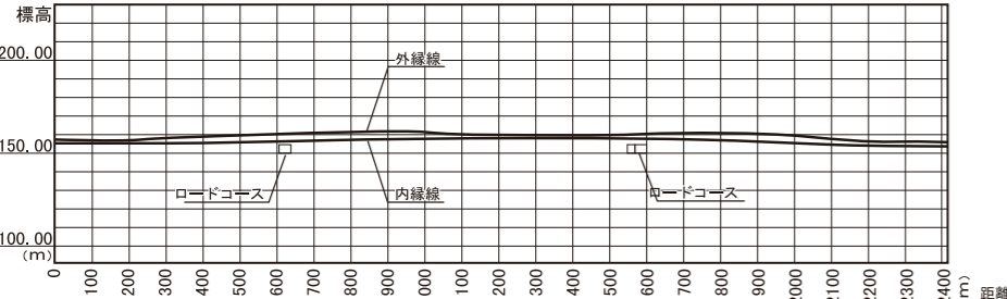
オーバルコース縦断図
